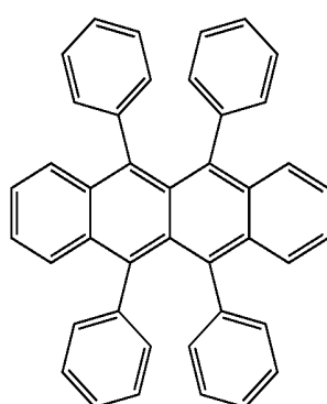
Rubrene
