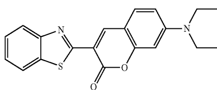
Coumarin 6
