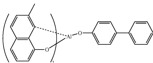
BAlq
